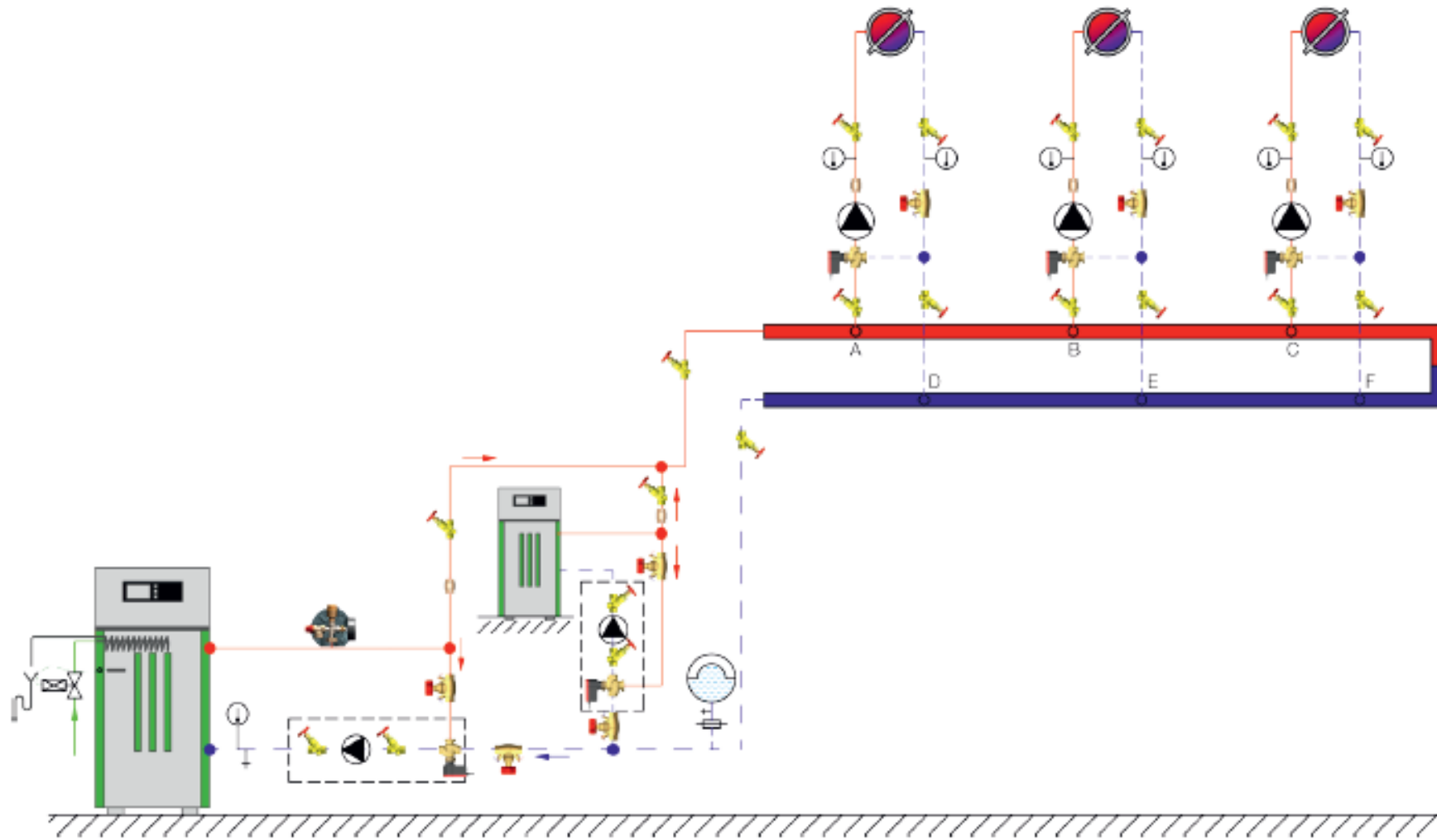
3.1.8./1. ábra: Nyomáskülönbség nélküli osztó-gyűjtő bypass-vezetékekkel
